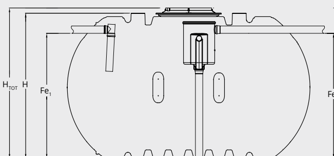
Fosses toutes eaux Carat XL super renforcées
