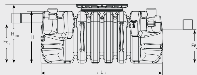
Bac à graisses 200 litres
