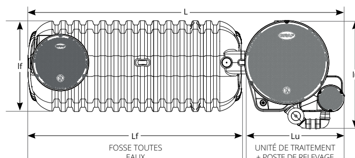
easyCompact 5 et 6 EH sortie haute avec poste de relevage
