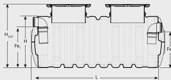
Bac à graisses 500 litres
